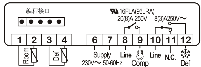
XR04CX - 压缩机输出瞬时最大电流 20A 或 8A
